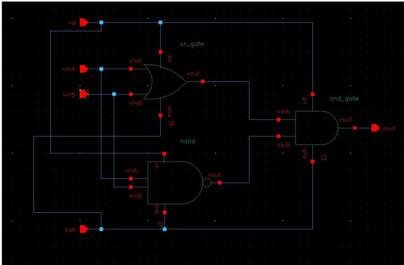
Xor gate Schematic
