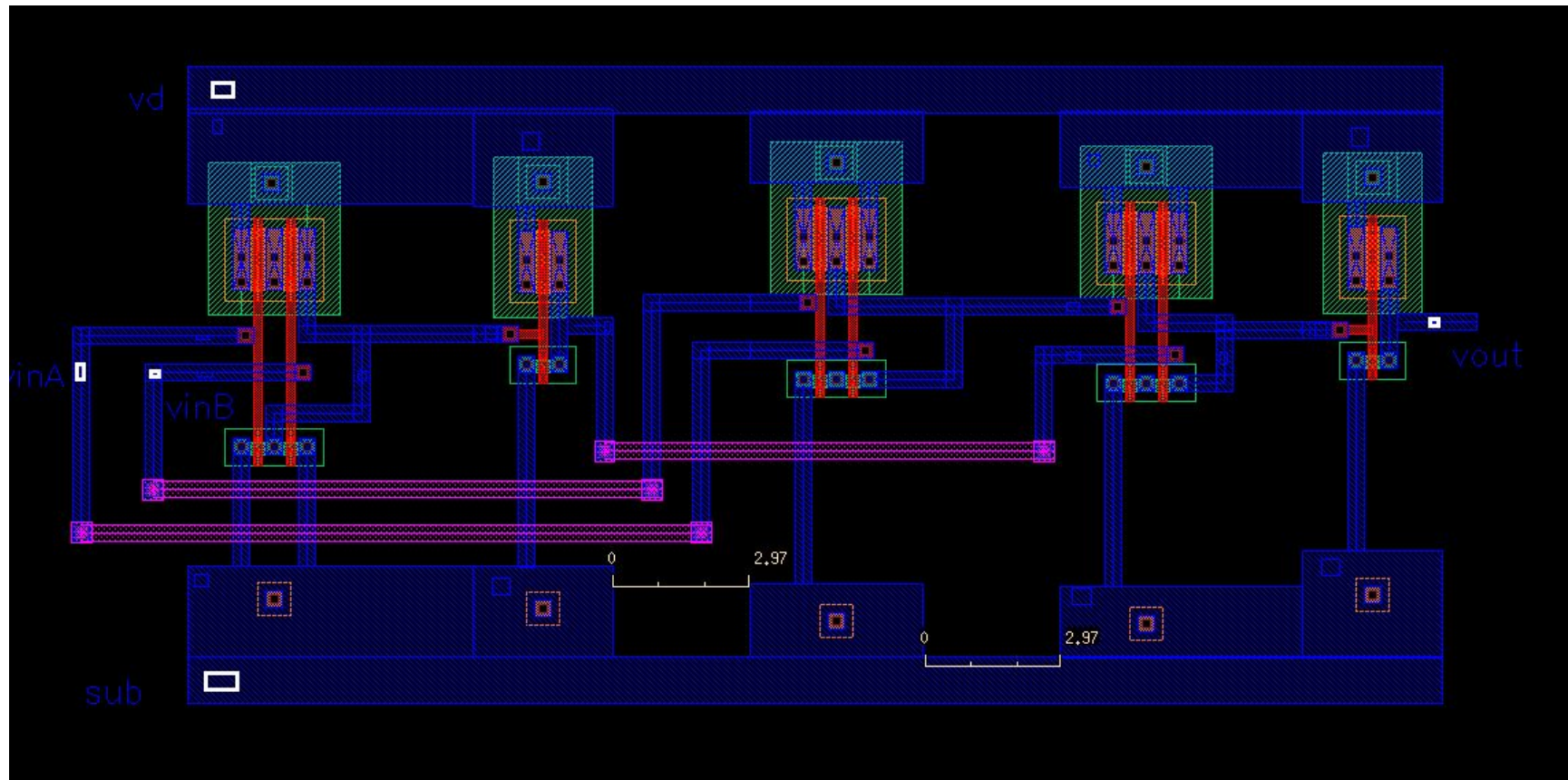
Xor gate Layout
